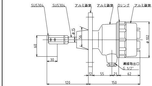
PRL-500N 型 耐荷重タイプ
