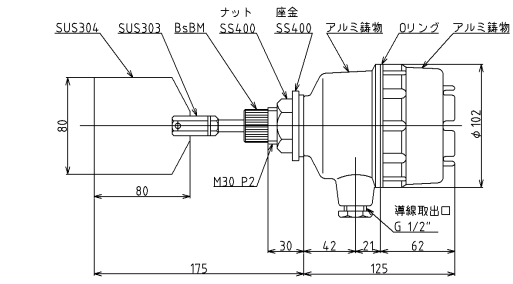
PRL-200 型 耐熱タイプ
