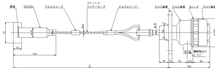
PRL-100EA/100EC 型 延長軸付固定式
