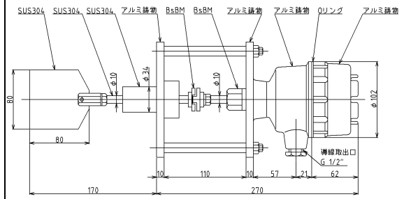
PRL-500 型 耐荷重タイプ
