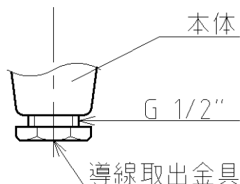
導線取出口
