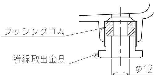
導線取出口(断面図)
