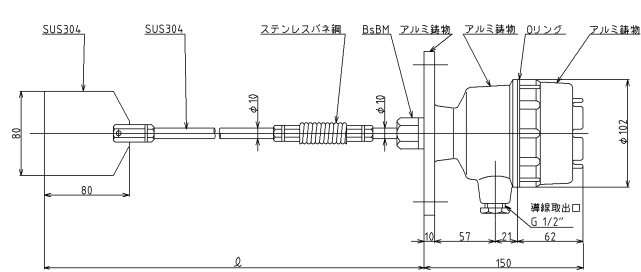
PRL-100EB/100ED 型 延長軸付伸縮式
