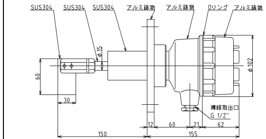
PRL-500N 型 耐荷重タイプ
