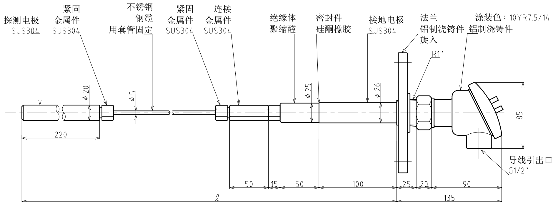
端子图
